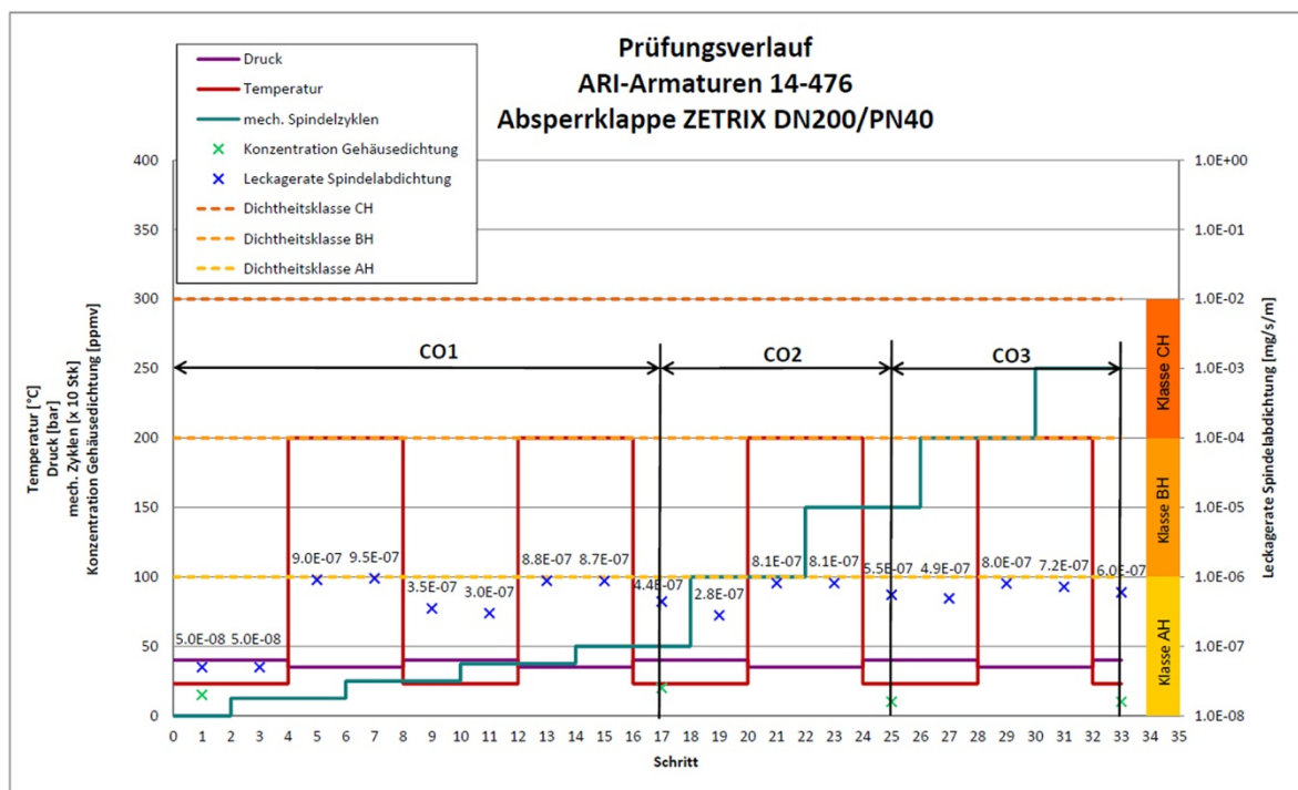
Abb. 3: Amtec-Prüfbericht Nr.: 302 586 2/- Beilage 15 – Prüfungsverlauf und Ergebnisse EN 15848-1 [3] [5]
