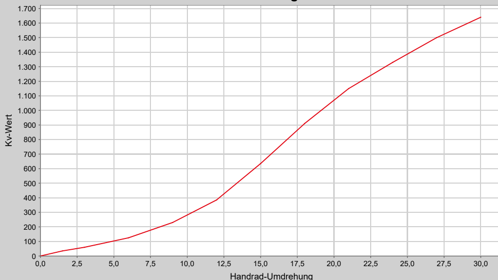
Kvs-Kennlinien-Diagramm
