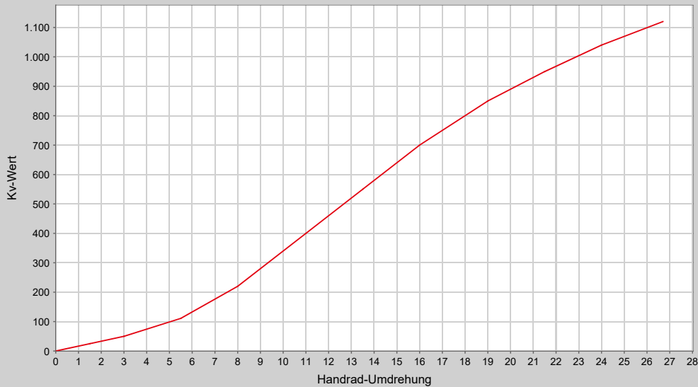
Kvs-Kennlinien-Diagramm
